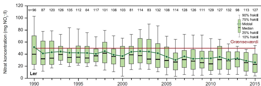
Figur 4.10. Udviklingen i det iltholdige grundvands nitratindhold i LOOP-oplande med sand (LOOP 2 og 6) og ler (LOOP 1, 3 og 4) vist som boksdiagrammer for hvert prøvetagningsår i perioden 1990-2015. Antallet af analyser er angivet for hvert år samt grænseværdien (kravværdien) for nitrat i grundvand og drikkevand.
